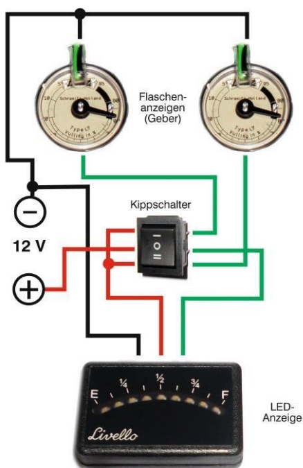
Schaltung 2-Flaschensystem
